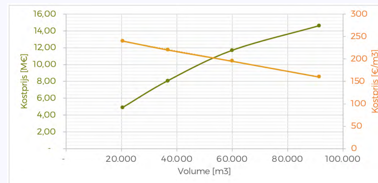
Figuur 2: Overzicht kostprijs van verschillende Ecovaten
